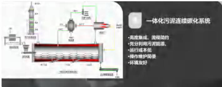
一体化污泥连续碳化系统工艺原理示意
